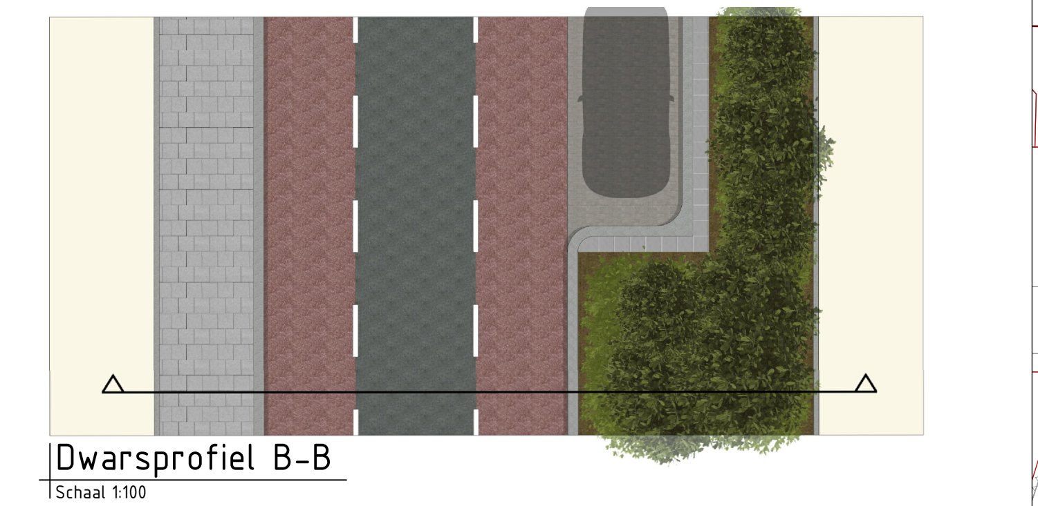
Dwarsprofiel B-B Schaal 1:100
