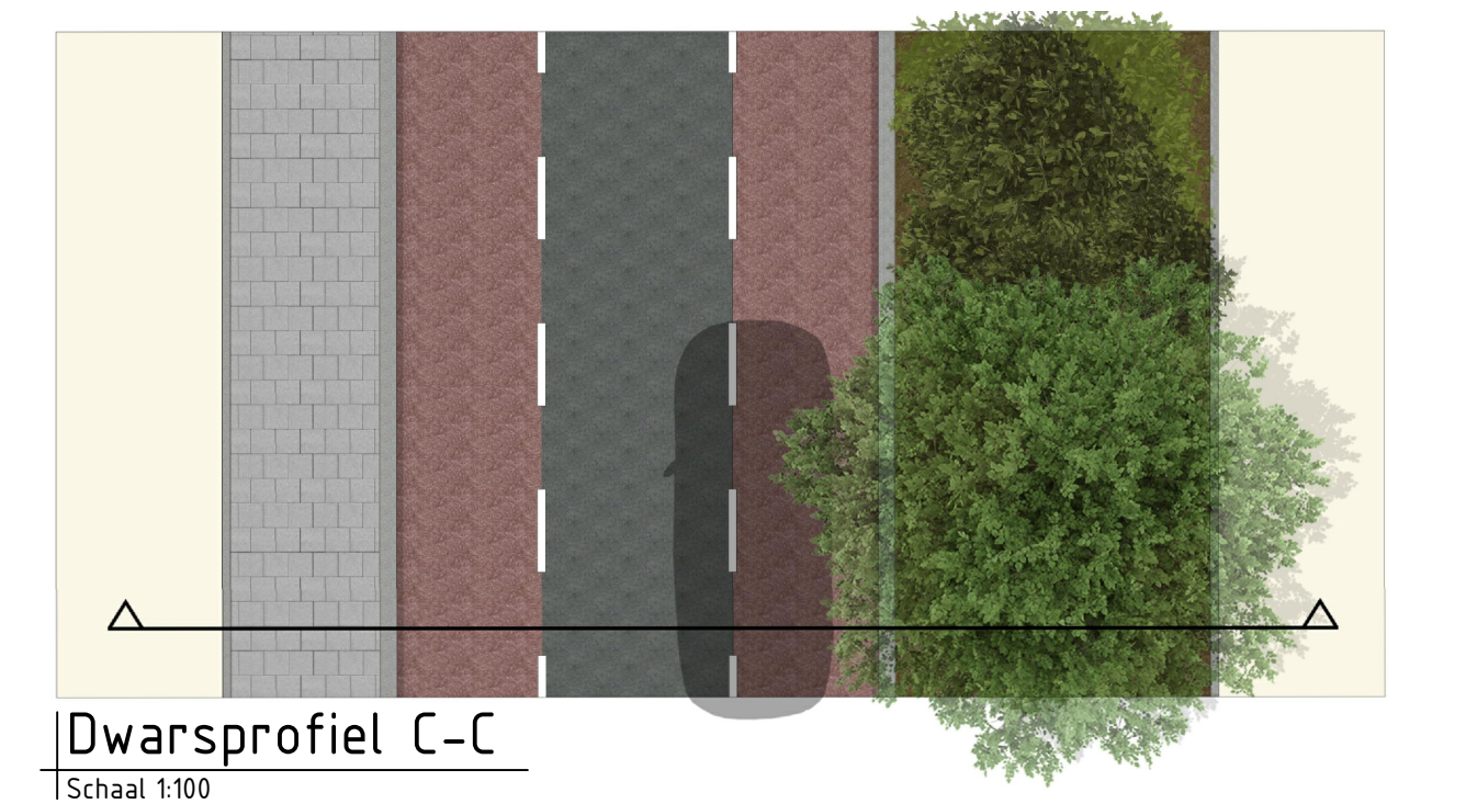
Dwarsprofiel C-C Schaal 1:100
